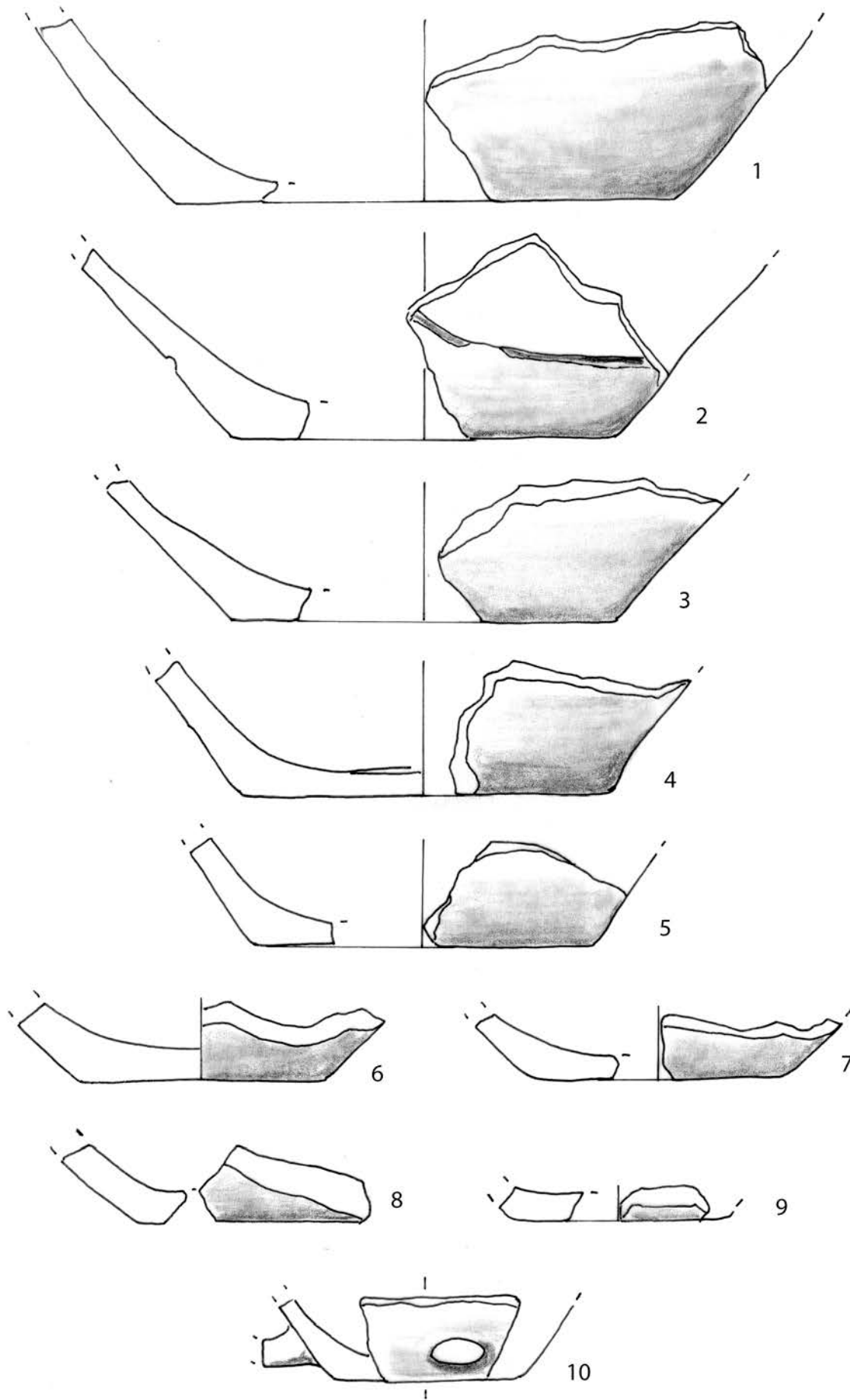
Fig. 99. Fondi. Scala 1:3.
