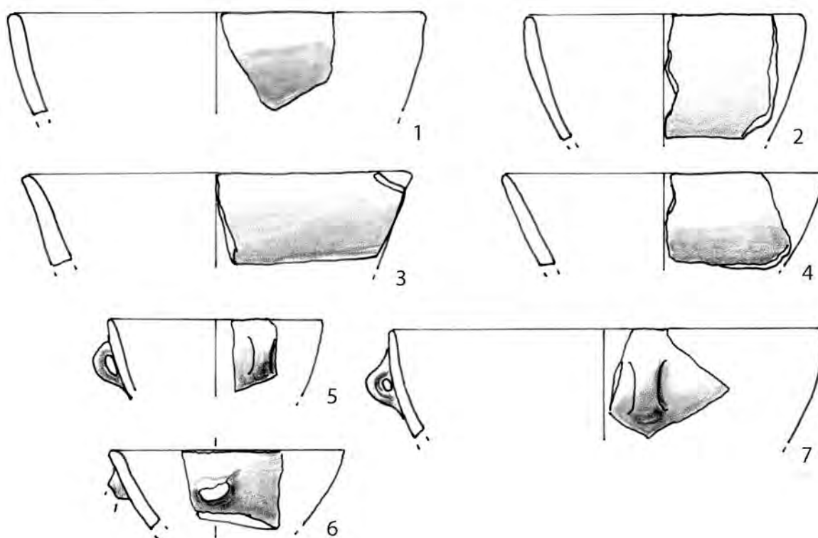
Fig. 65. Mursia B14. Scodelle. Scala 1:3.
