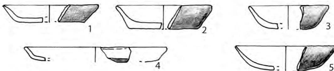
Fig. 62. Mursia B14. Tazze-Ciotole (TC). Scala 1:3.
